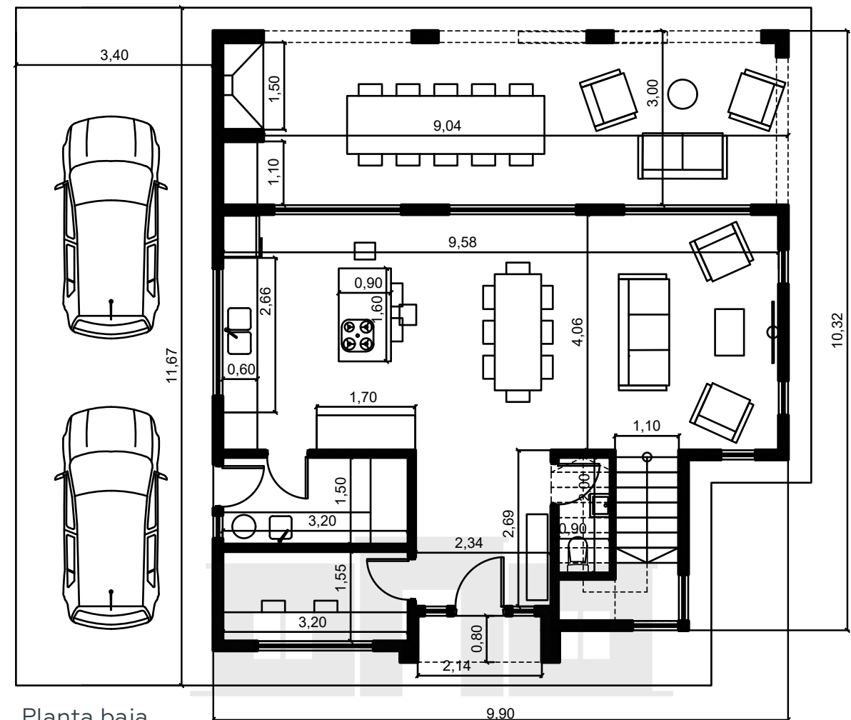
Planta baja
