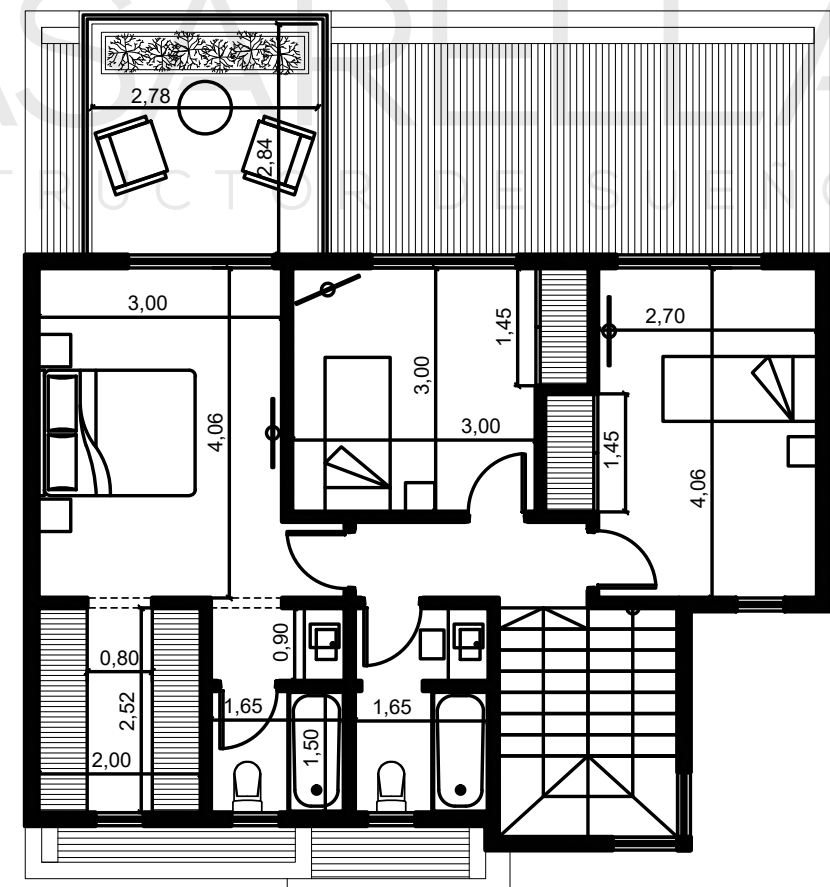
Planta alta
